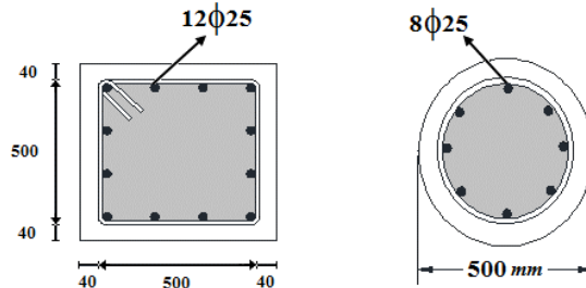
شکل ۵: جزئیات مقاطع ستون‌های مورد بررسی
