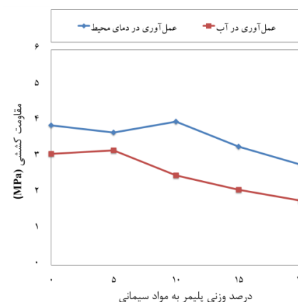
ب - مقاومت کششی ۱۴ روزه
