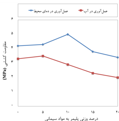
ج - مقاومت کششی ۲۸ روزه
