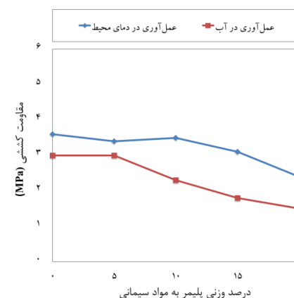
الف - مقاومت کششی ۷ روزه
