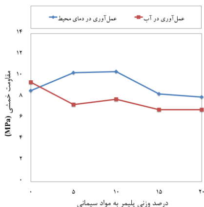
ج - مقاومت خمشی ۲۸ روزه
