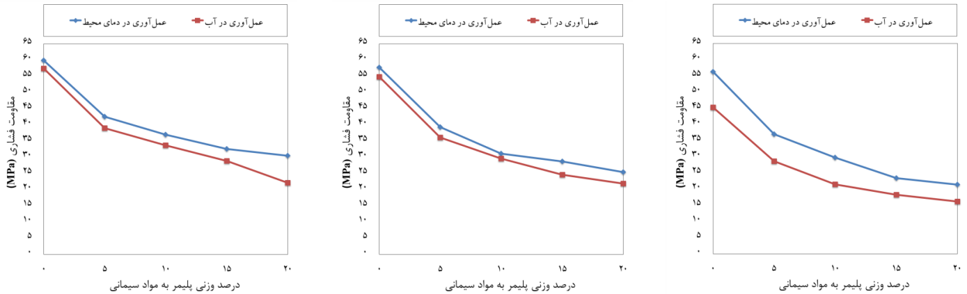
ج- مقاومت فشاری ۲۸ روزه
