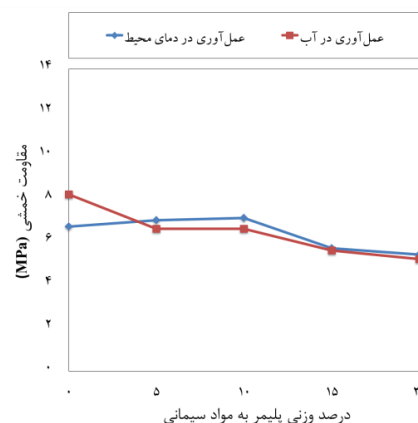
الف - مقاومت خمشی ۷ روزه
