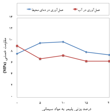
ب - مقاومت خمشی ۱۴ روزه
